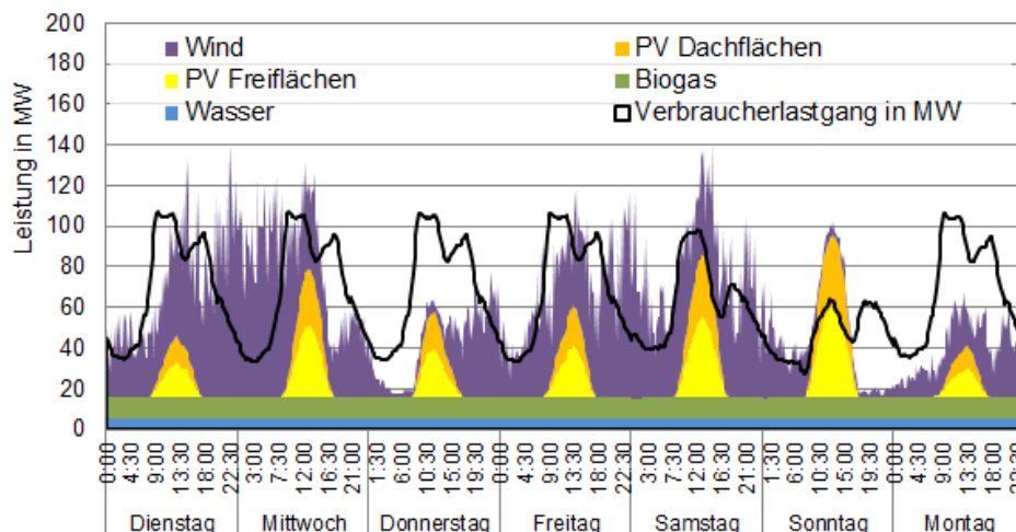
Abbildung 7.6: Strom-Lastanganalyse für 04. bis 10. Februar, nach einem angenommenen Ausbau der Windkraft um eine Erzeugungskapazität von 300.000 MWh/a
