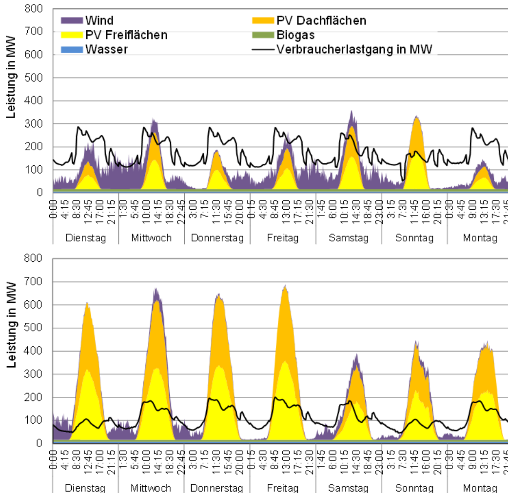
Abbildung 7.4: Strom-Lastanganalyse für das Zieljahr 2024. Oben für den Zeitraum 04. bis 10. Februar, unten für den Zeitraum 01. bis 07. Mai
