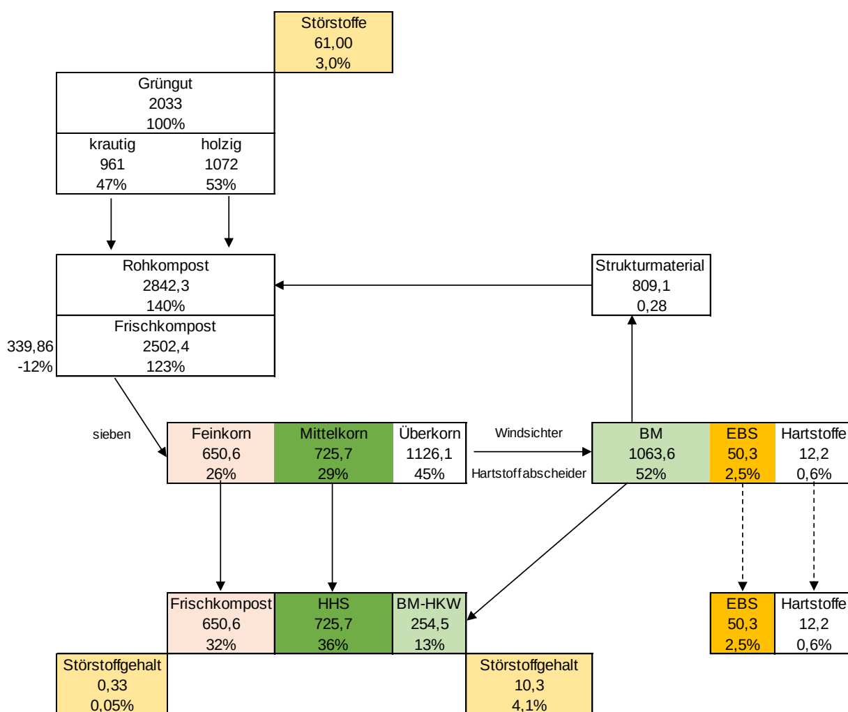
Abbildung 7.9: Stoffmassenbilanz am Beispiel einer Zentralanlage in Langerringen
