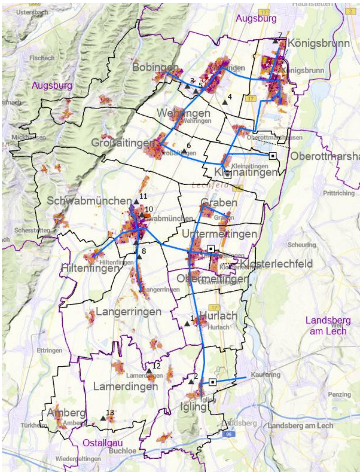
Abbildung 7.12: Wärmenetzkonzept für Nord und Süd. Abgebildet: Zweiteilige Versorgung ohne Verbindungsleitung zwischen Kleinaitingen und Graben.
